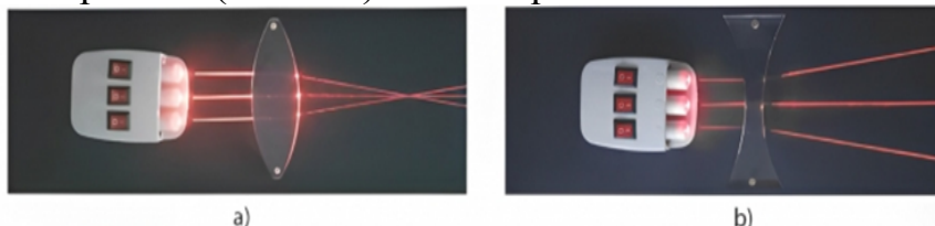
Hình 8.3 Đường truyền của ba chùm sáng hẹp, song song qua thấu kính hội tụ (a) và qua thấu kính phân kì (b)
